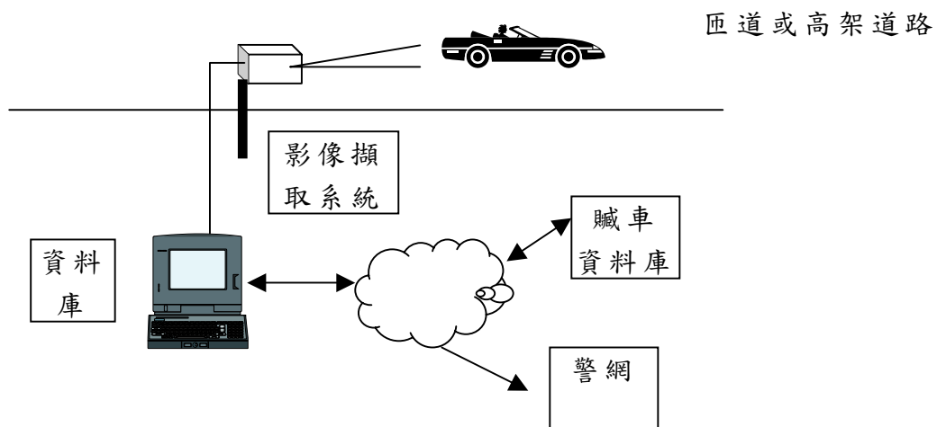
圖十： 贓車自動查緝系統
